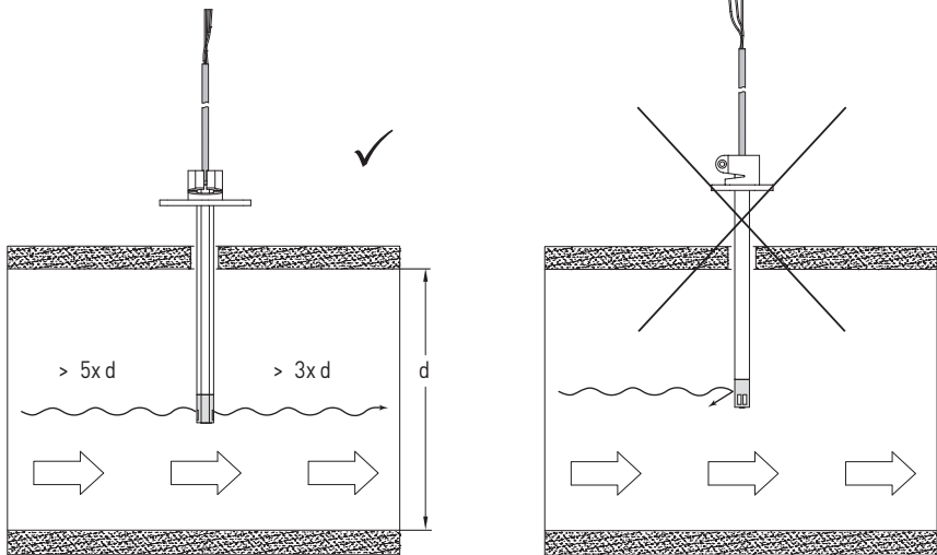
Einbauschema
