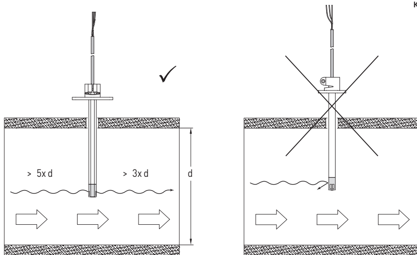
Схема монтажа
